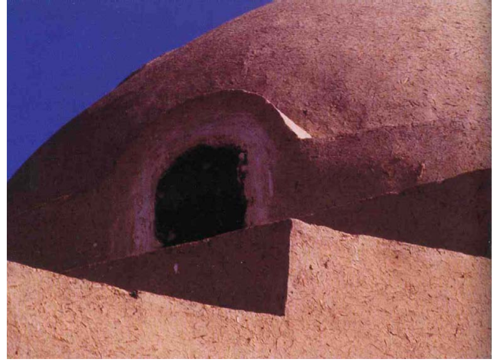
منزل ستوبلير بالأقصر و تظهر الدعائم المتدرجة عند قاعدة القبة.
