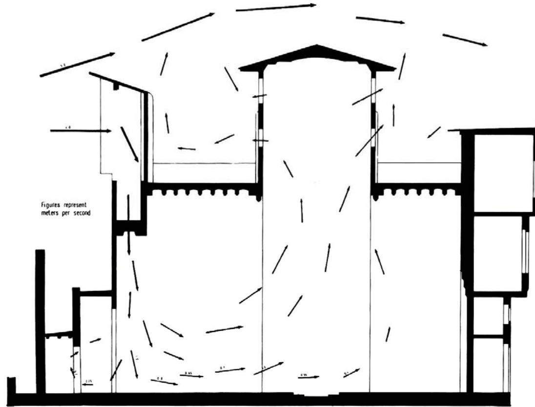
دراسة لحركة الهواء في بيت محب الدين أجريت بواسطة فريق من الجمعية المعمارية في لندن و شارك فيها عمر الفاروق . حيث تدخل الرياح الشمالية الشرقية الساندة الي الملفف و تبرد المساحة الداخلية فيرتفع الهواء الساخن و يخرج من الشخيشة الموجودة بأعلى القاعة.
