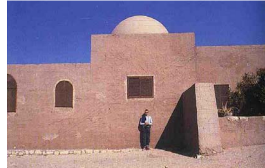
منزل ستوبلير بالأقصر و تظهر الدعائم المتدرجة عند قاعدة القبة.
