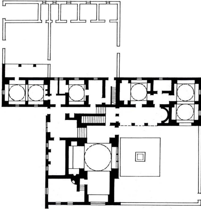
مخطط منزل قليني - 1945 - واحد من أكثر تصميمات فتحي براعة. الفصل الواضح بين المساحات العامة والخاصة تمت مراعاته حيث يمكن الوصول السهل إلى الفناء المشترك (الجزء السفلي يمين) مع وجود ممر مسقف كمنطقة وسيطة.
