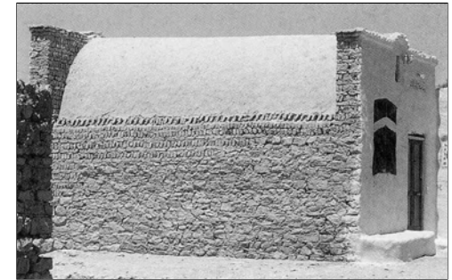
منزل معاصر في أبو الريش يظهر القبو الذي تعلمه فتحى في أربعينات القرن العشرين . بعد بناء الحائطين الجانبيين و الحائط الخلفي يتم بناء القبو بوضع كل صف من الطوب بميل عن الصف السابق و في النهاية يتم بناء الحائط الامامي.
