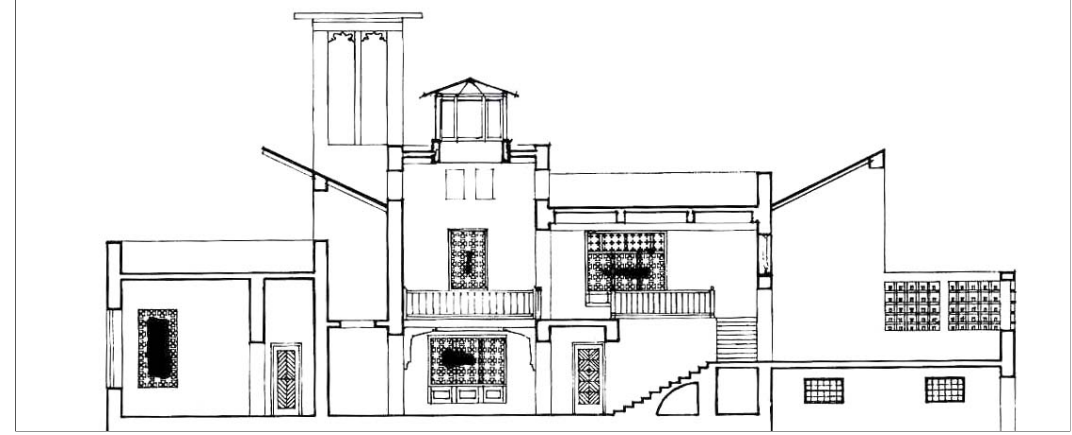
قطاع في منزل نصيف بجدة بوضوح القاعة والملفك و يحتوي المنزل على اجمل أعمال الخشب المزخرف في كل مبانيه فتحتي.
