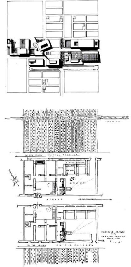
المخطط العام و مخطط لوحدة سكنية في البرنامج الإسكان العراقي . بالرغم من اختلافه عن مشاريعه الأولى فإن هذا التصميم يسمح للسكان بالوصول المباشر إلى الحقول الزراعية و هي صفة للقرى العراقية التي زارها فتحي.
