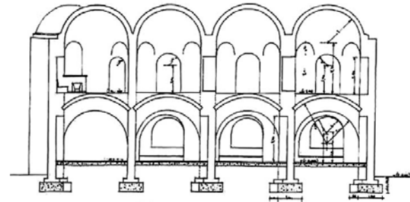
قطاع في استراحة شركة التعدين.
