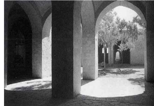
مدرسة فارس تتم صيانتها بعناية ويلاحظ إن كل فصل يطوه قبو للتهوية الطبيعية.
